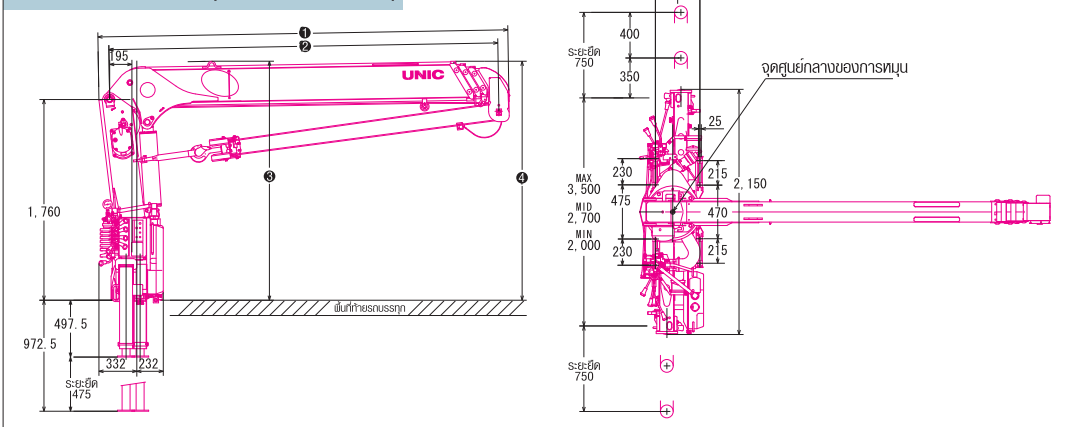
แบบร่าง: UR-V344 (หน่วย : มิลลิเมตร)
